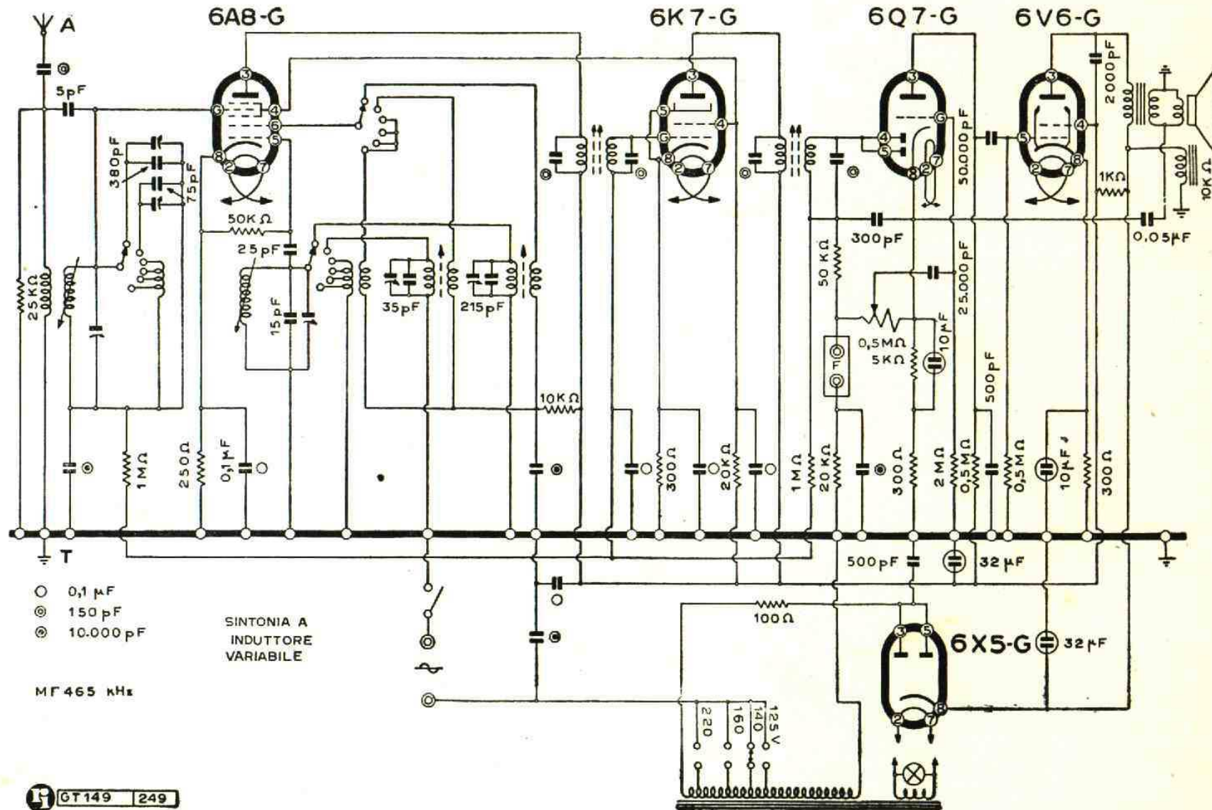
Lo schema elettrico del mod. 526 (I serie)
